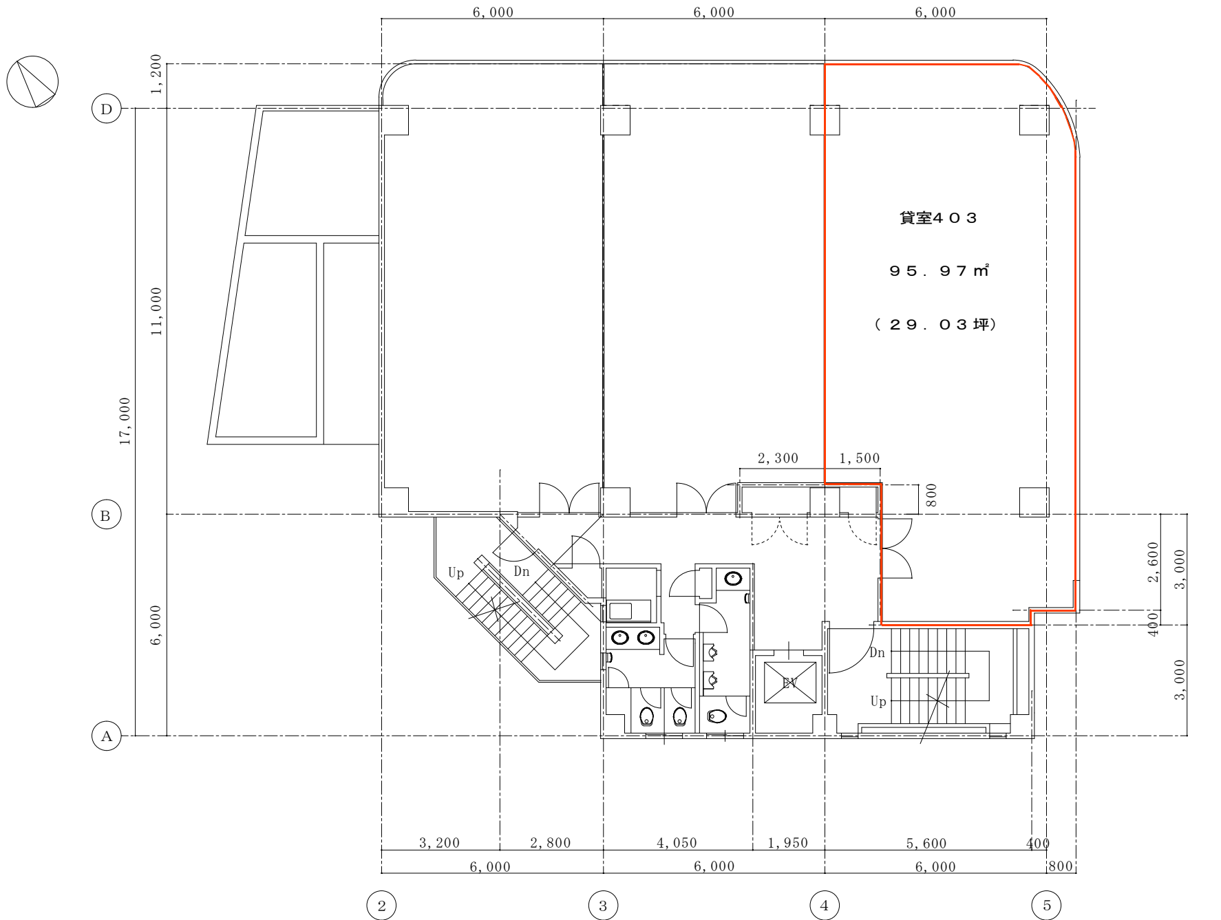
DO!野並 4階 平面図
