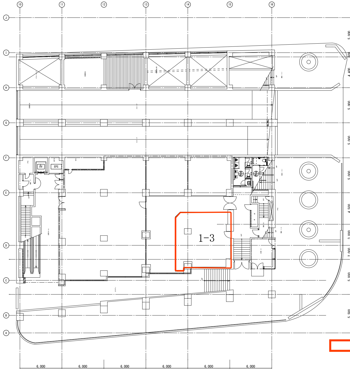
チカシン池下 1階 平面図
