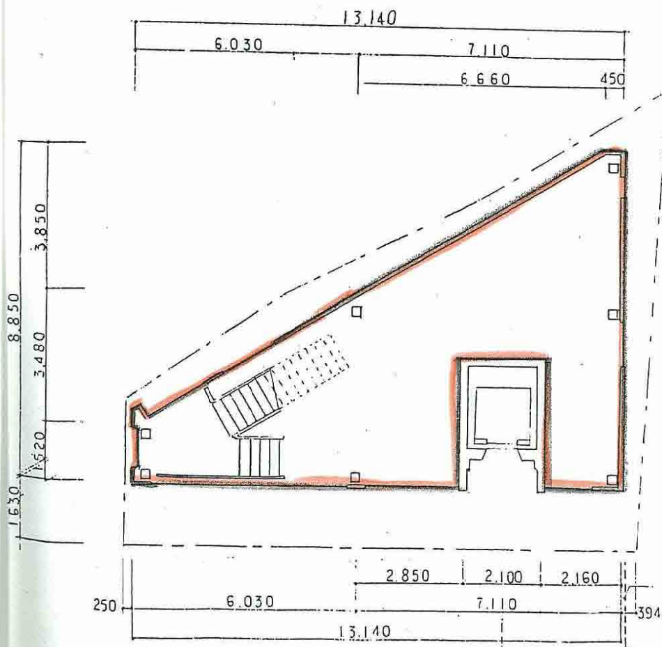
1階平面図
